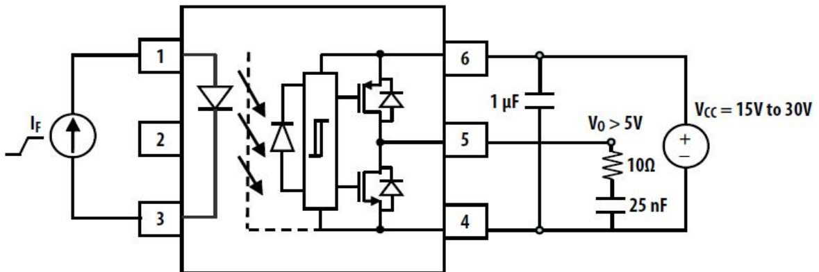
图例 18-IFLH 测试电路
