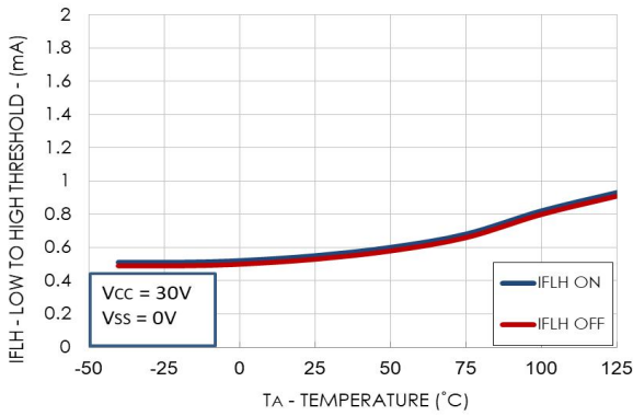
图例 7-阈值电流从低到高与工作温度曲线图 Fig.7 IFLH vs. Temperature
