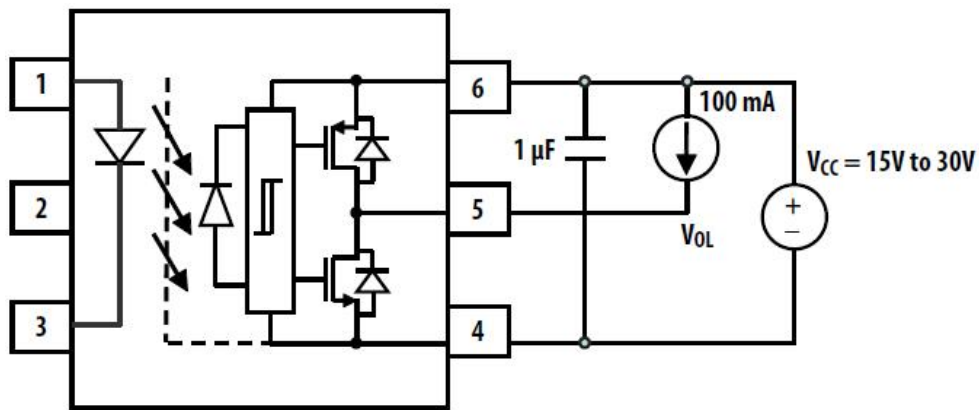
图例 17-VOL 测试电路
