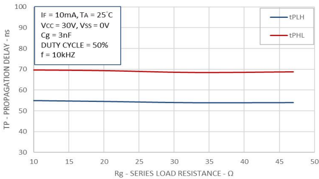
图例 11-传输延时与负载电阻曲线图 Fig.11 Propagation Delays vs. Rg
