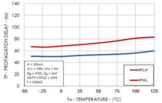
图例 10-传输延时与工作温度曲线图 Fig.10 Propagation Delays vs. Temperature
