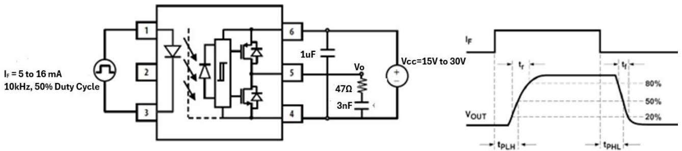
图例 20-传输延时测试电路及波形图 Fig.20 tPHL, tPLH, tr and tf Test Circuit and Waveforms
